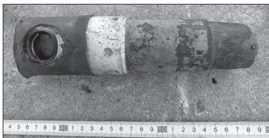
Прицел для бомбометания Ил-4 (фрагмент)
